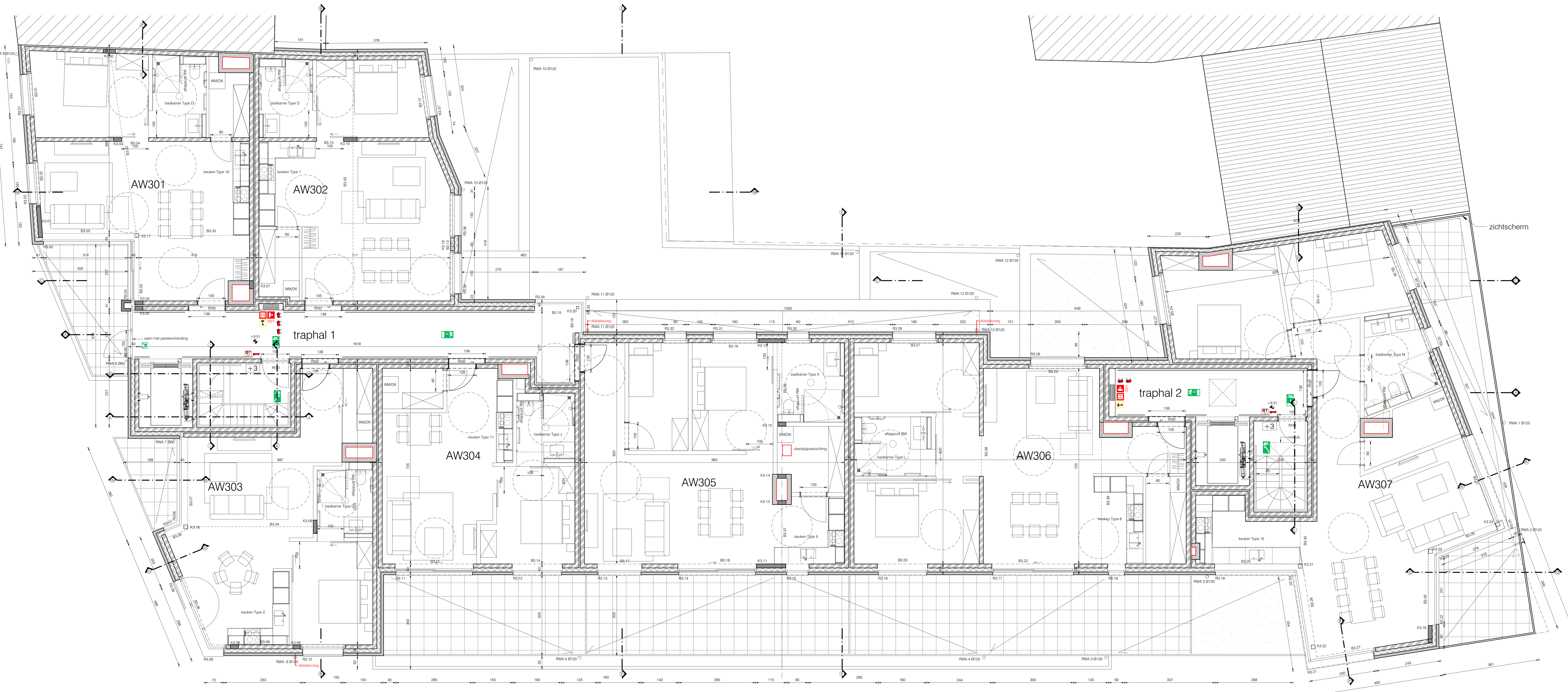
grondplan verdieping +3 schaal 1:50
