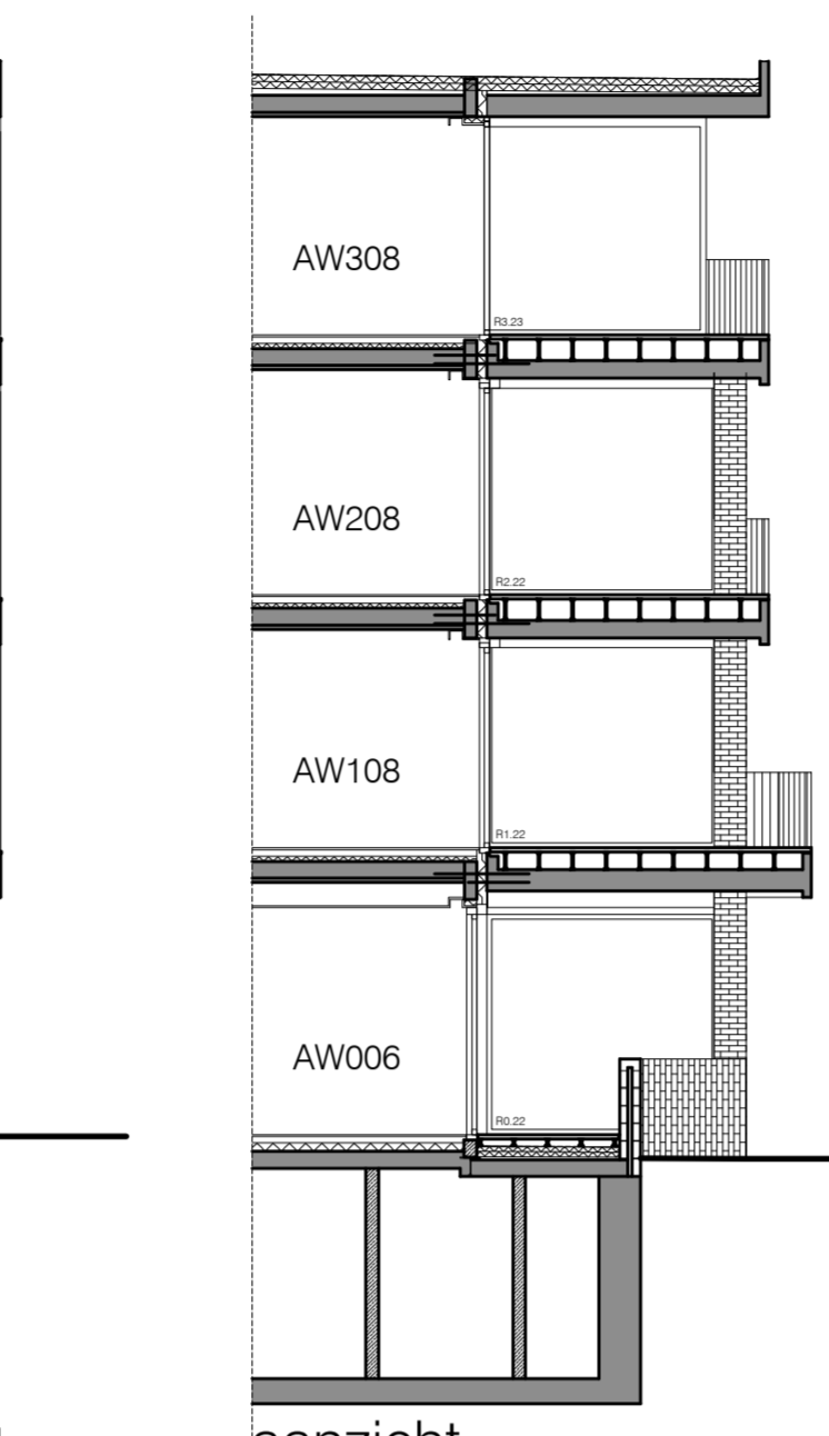
aanzicht snede Q schaal 1:100
