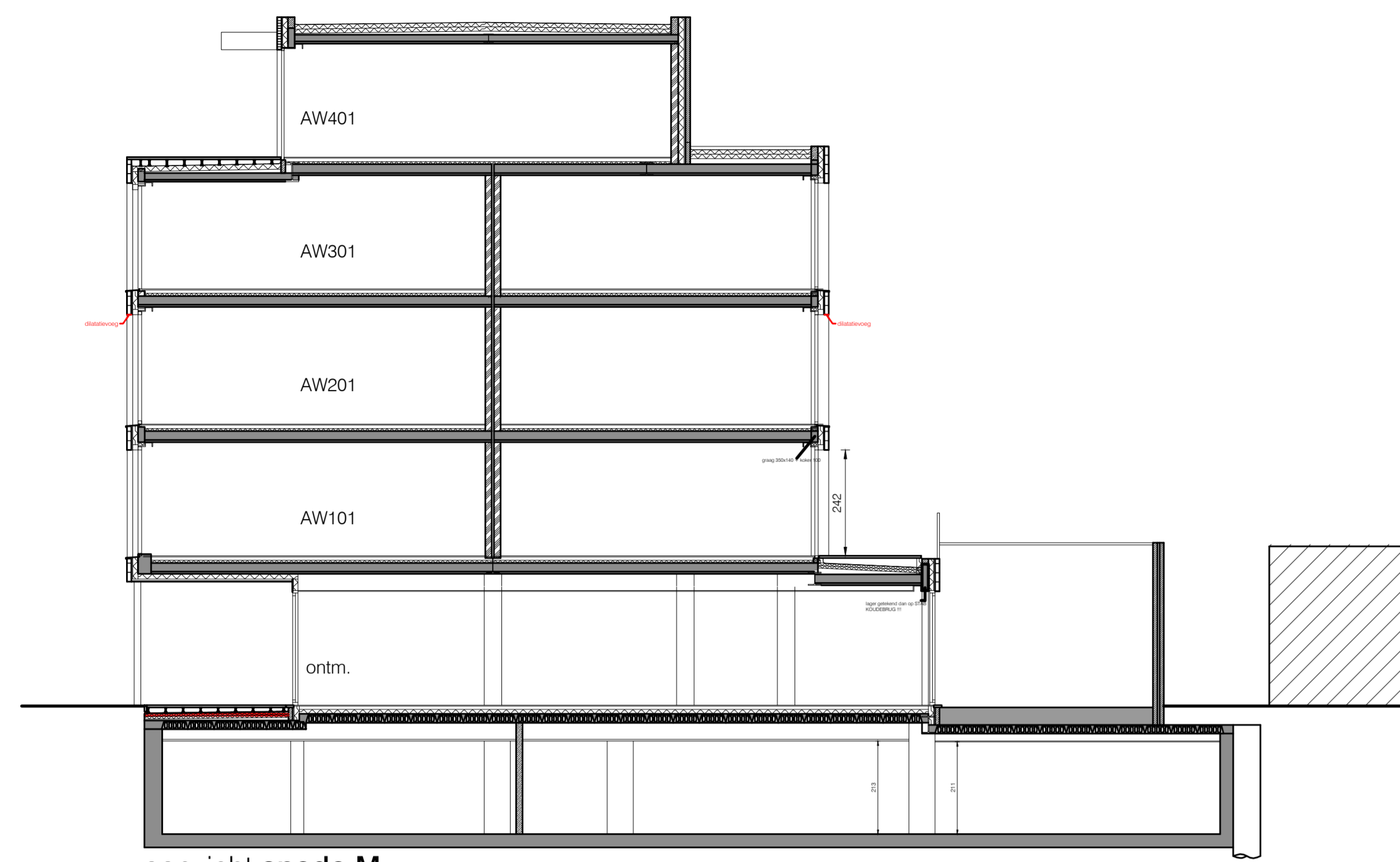
aanzicht snede M schaal 1:100
