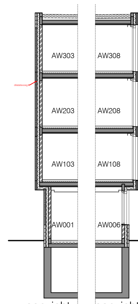
aanzicht snede O schaal 1:100
